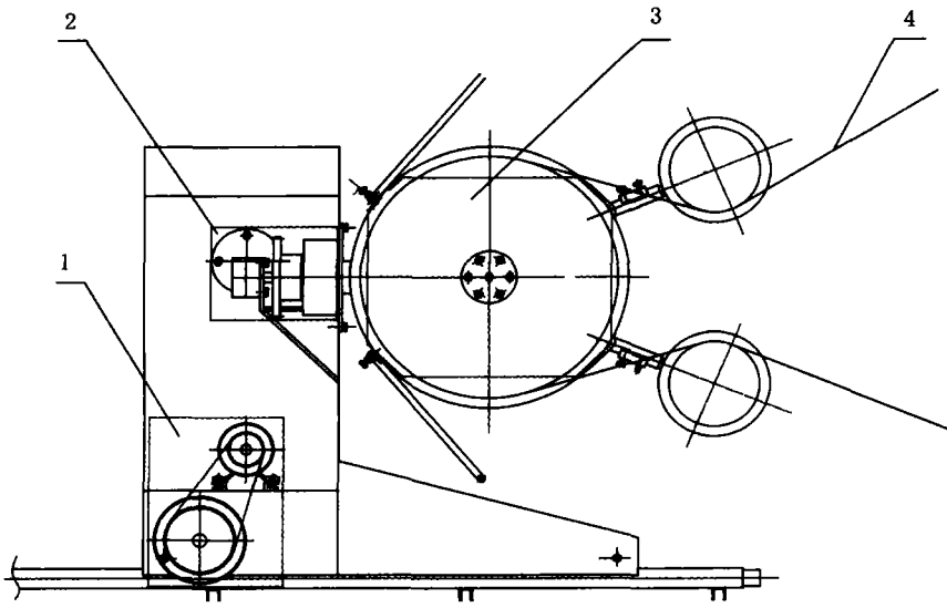
1-行走机构 2-转角机构 3-动力机构 4-串珠绳 图2 金刚石串珠锯结构示意图
