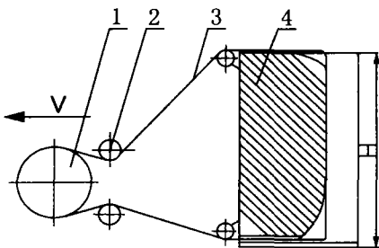
1- 主驱动轮 2- 导向轮 3- 串珠绳 4- 石材 图1 金刚石串珠锯工作原理图
