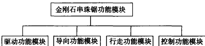
图3 串珠锯的功能模块
